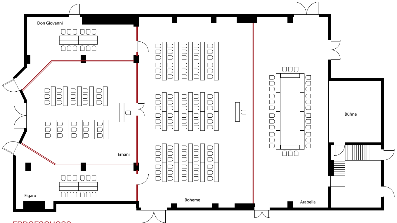
ERDGESCHOSS
